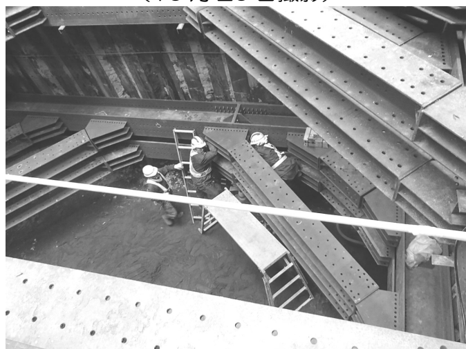
切梁等で補強しながら掘削を進めていきます (12月12日撮影)
