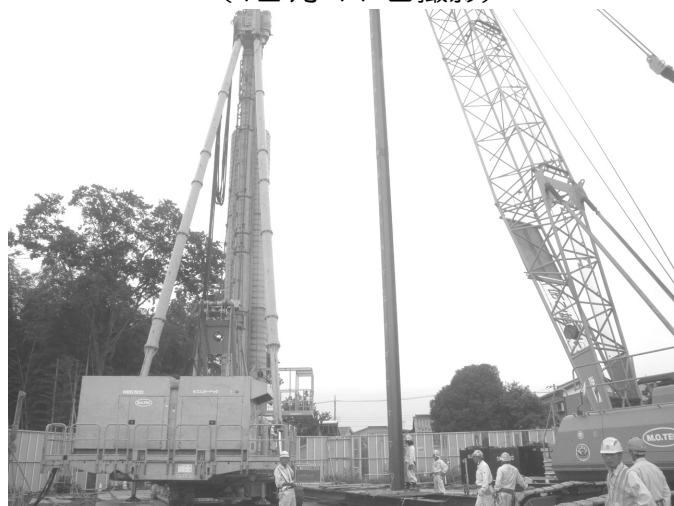
立坑のため長さ 24.5 メートルの H 鋼を埋め込みます (9月10日撮影)
