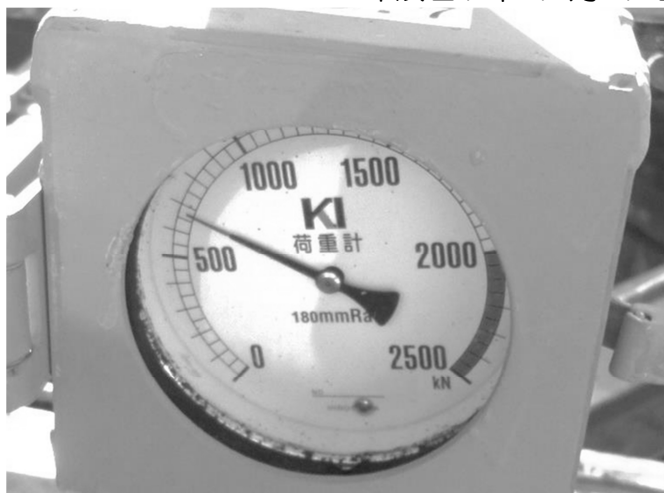
荷重計で切梁にかかる土圧を計測しています 写真は約 70 トン！（12 月 17 日撮影）
